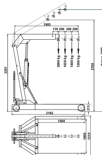
3 Żuraw o nośności 2 tony, z osią przewodzącą, łatwy w manewrowaniu. Z równoległym podwoziem do pracy z paletami.
