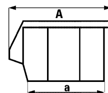
A = vonkajšia dĺžka, a = vnútorná dĺžka
