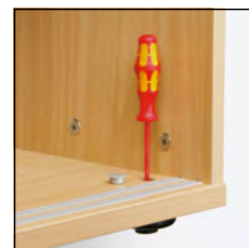
Nastavitev višine skozi dno omare
