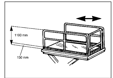
Op aanvraag: balustrade – met zijdelings scharnier
