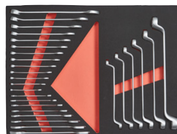
27 delen – ring- en steeksleutels
