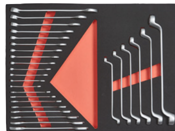
27 elementi – chiavi ad anello e chiavi fisse
