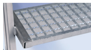
Plate-forme et marches en caillebotis galvanisé à chaud
