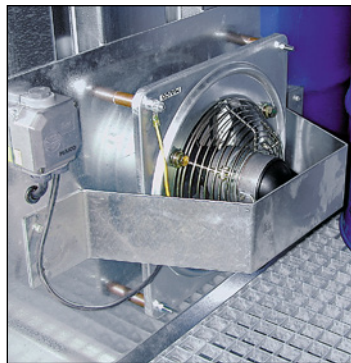
Ventilation antidéflagrante
