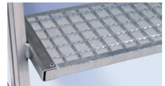
Plattform und Stufen aus Gitterrost, feuerverzinkt
