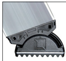
Bewegliches Gelenk mit patentierter 2-Achsen-Neigungstechnik
