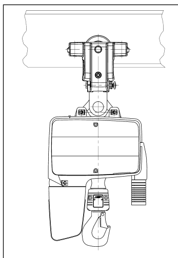
Rollfahrwerk
