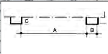
Dimensions passages pour fourches (dimensions intérieures): A = écart entre passages pour fourches, B = largeur des passages pour fourches, C = hauteur des passages pour fourches
