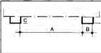
Abmessungen der Einfahrtaschen (Innenmaße): A = Einfahrtaschenabstand, B = Einfahrtaschenbreite, C = Einfahrtaschenhöhe
