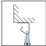
Hakenleiste unter Sturz
