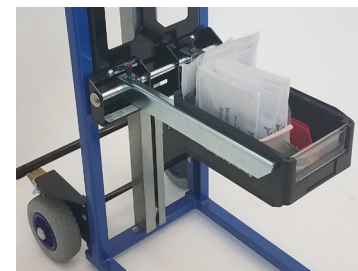
11 | Kastengabeln für Materialheber und Hubkarre
