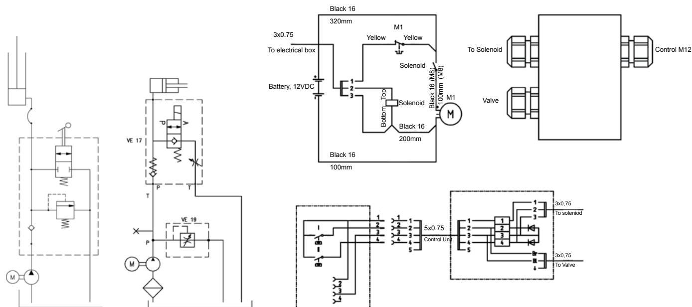
Akutoitel töötava hüdraulikamootori elektriskeem
