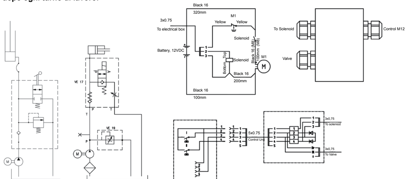
Schema elettrico, unità di alimentazione a batteria
