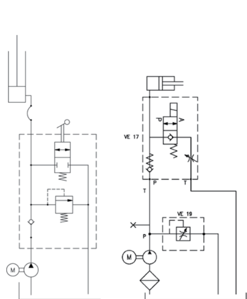
Schéma hydrauliky
