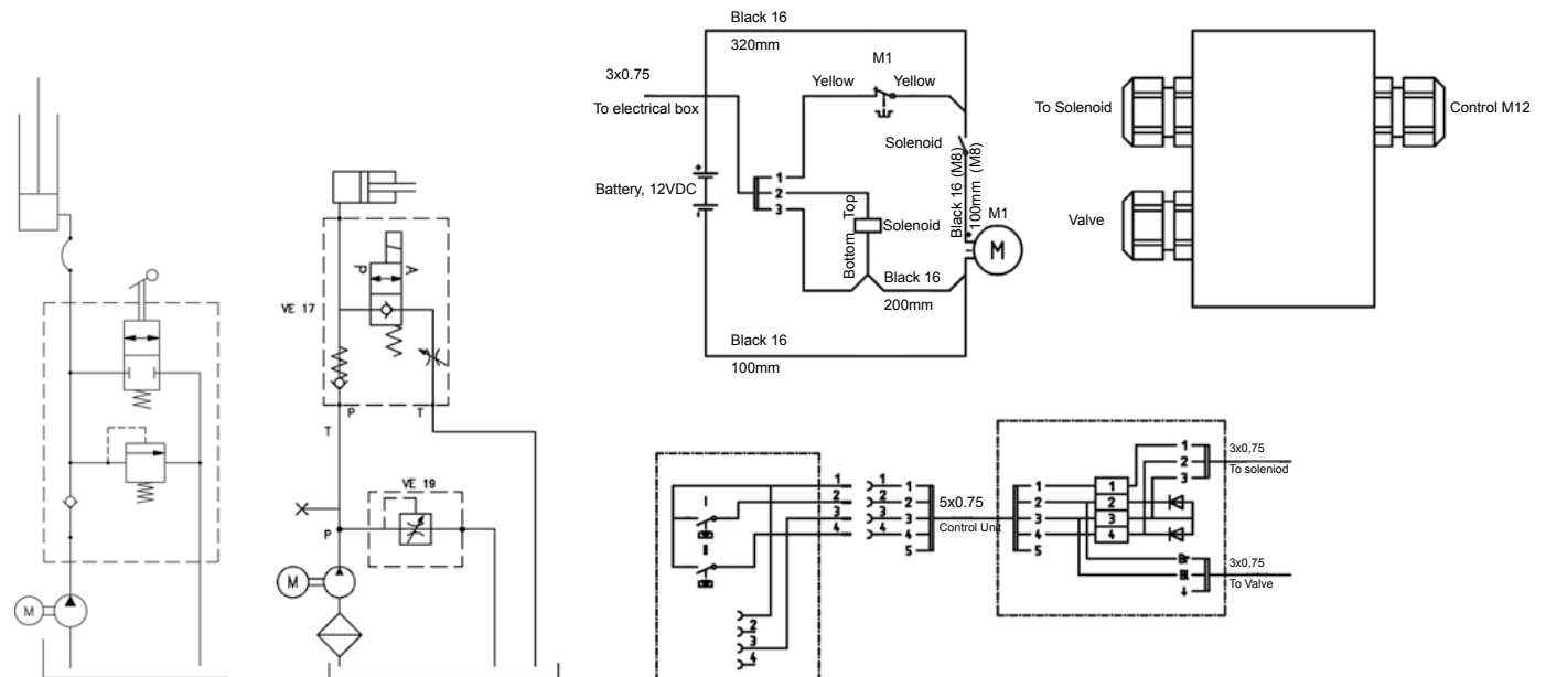
Esquema eléctrico, unidad de alimentación alimentada por batería
