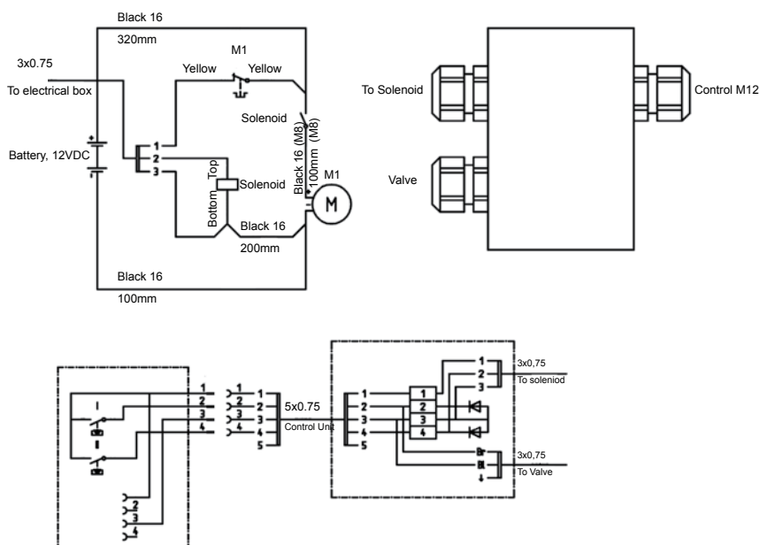
Schéma elektrického zapojení, pohonná jednotka s bateriovým napájením
