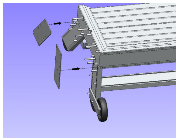
Knotenblech wieder montieren
