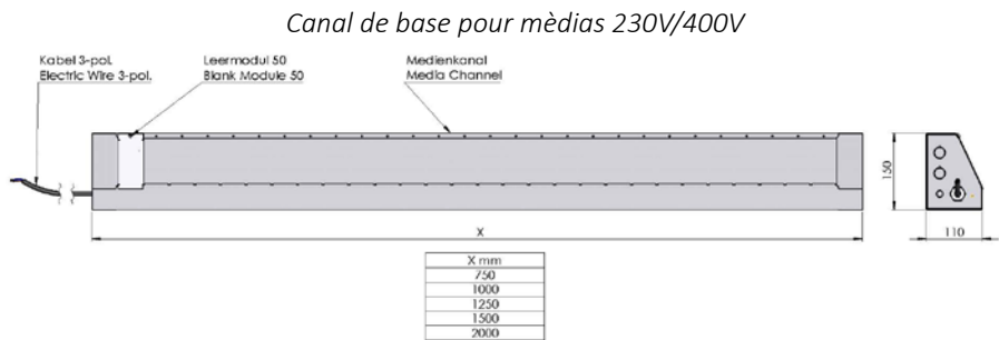
Illustration 1. Canal de base pour médias 230V et 400V avec couvercle aveugle et câble de connexion.
