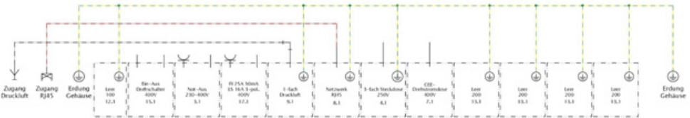
Referenzplan 400V
