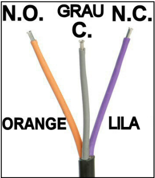
Abb. 5 Kontaktbelegung Signalkabel
