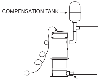
RÜCKSCHLAGVENTIL (automatische Pumpe)
