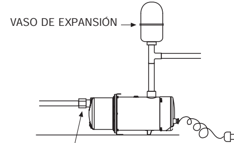
VÁLVULA DE RETENCIÓN (en la versión automática)
