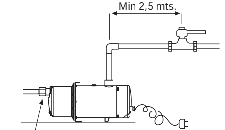
VÁLVULA DE RETENCIÓN (en la versión automática)
