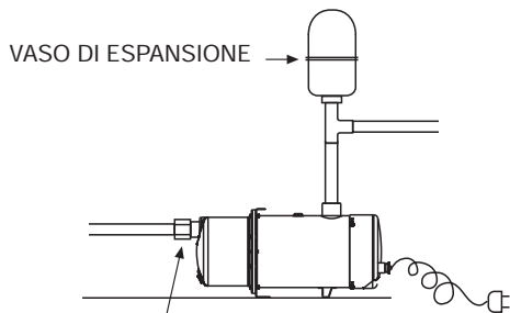
VALVOLA RITEGNO (nella versione automatica)
