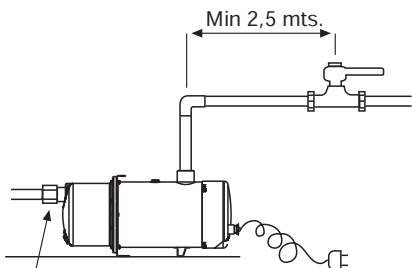
RÜCKSCHLAGVENTIL (automatische Pumpe)
