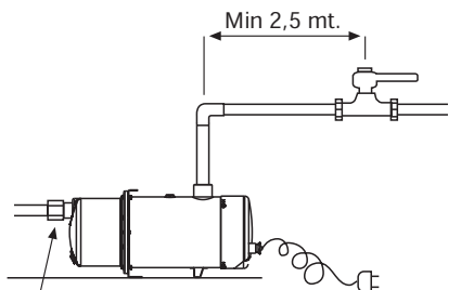
VALVOLA RITEGNO (nella versione automatica)
