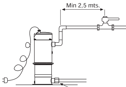
RÜCKSCHLAGVENTIL (automatische Pumpe)
