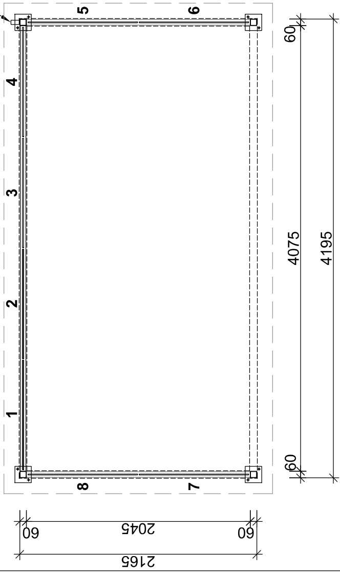
Grundriss
