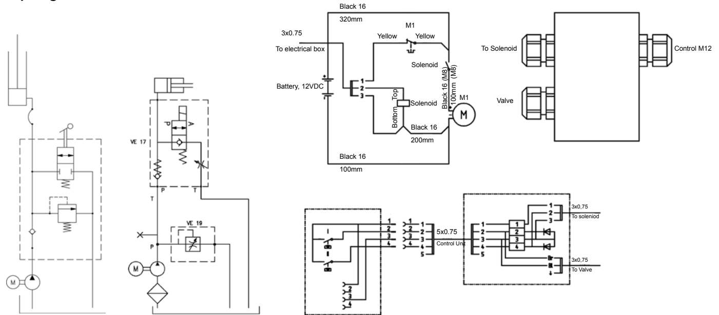
Schema idraulico
