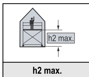
h2 max. Dopuszczalna maksymalna wysokość rusztowania wewnątrz budynków
