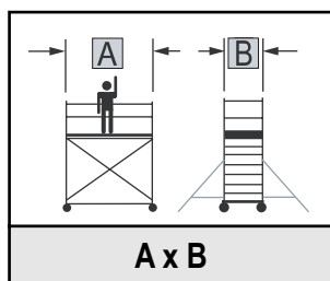
Longueur plancher x Largeur du cadre
