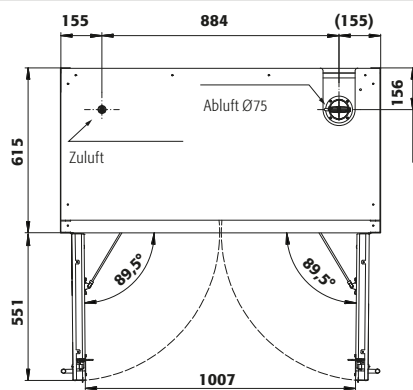
Draufsicht
