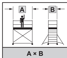
Tellingute pikkus × raami laius
