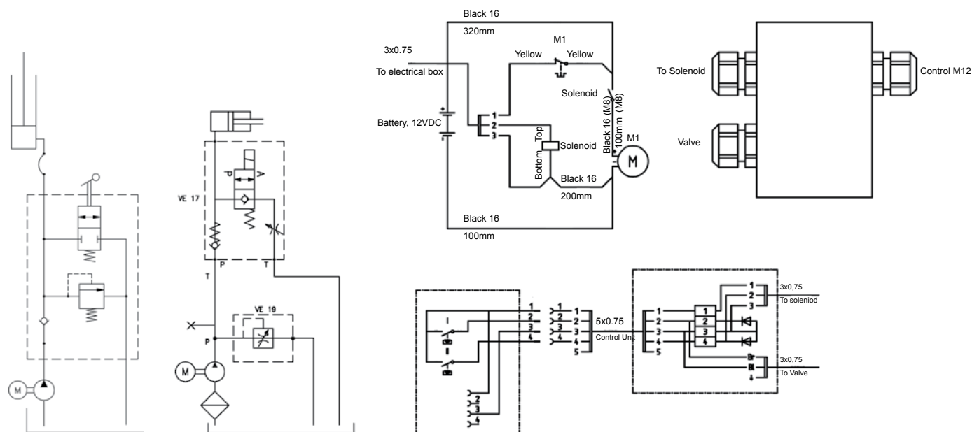
Hydraulikskema
