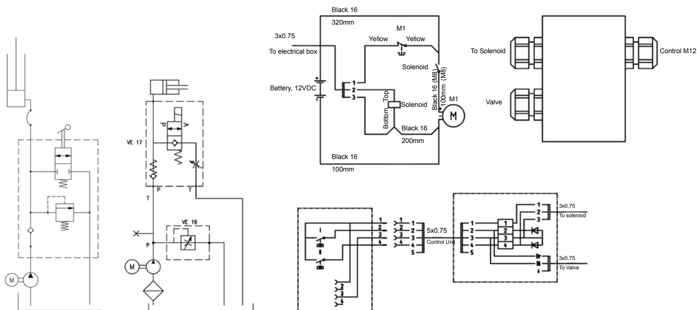
Hydrauliskema
