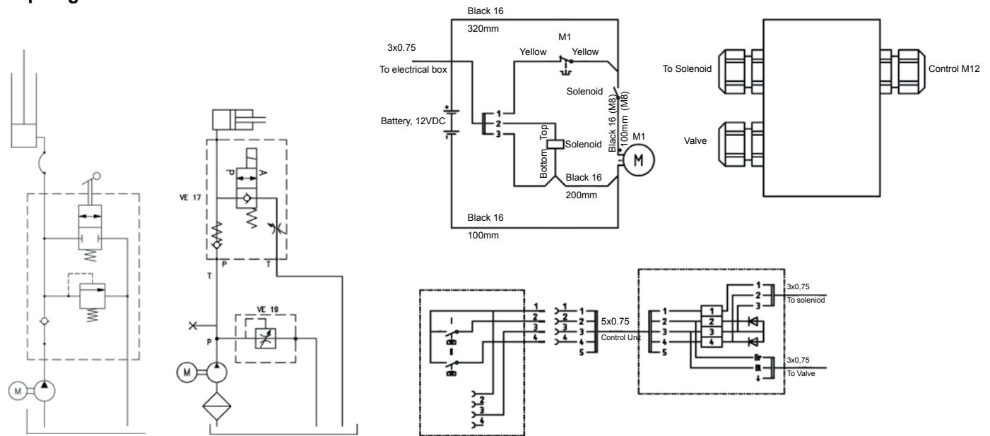
Schema idraulico
