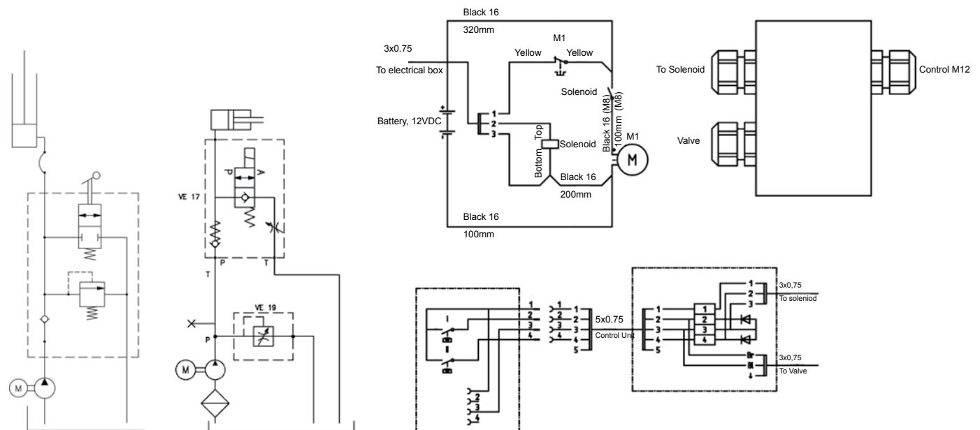
Esquema eléctrico, unidad de alimentación alimentada por batería
