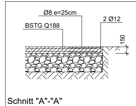
(Fertig-) Bodenplatte
