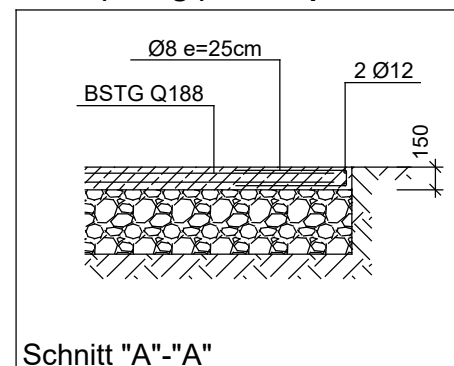
(Fertig-) Bodenplatte
