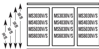
Anordnung für 120-cm-Querstreben
