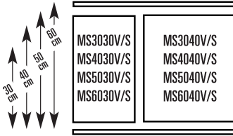
Innordning for 100 cm tverrstenger
