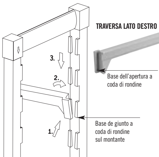
MONTARE LE TRAVESSA SUI MONTANTI
