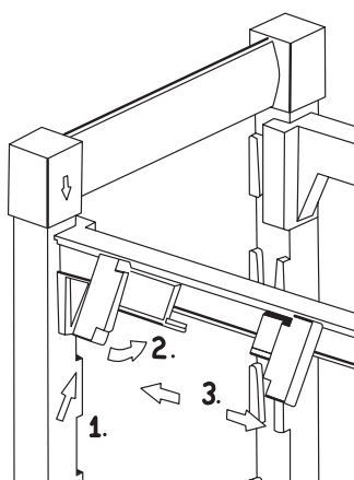
SNAPPVERBINDUNGEN DER QUERSTREBE
