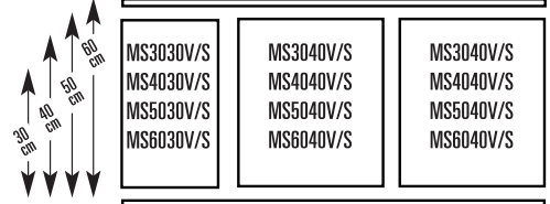
Innordning for 130 cm tverrstenger
