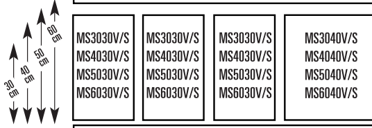
Innordning for 150 cm tverrstenger
