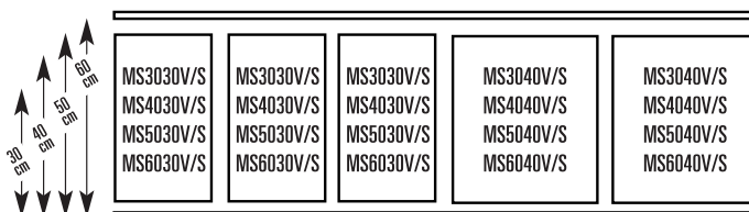
Disposición para traviesas de 170 cm
