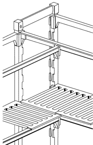
TVÄRSTAGENS MONTERING
