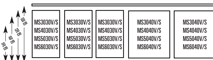
Indeling voor dwarsliggers van 170 cm
