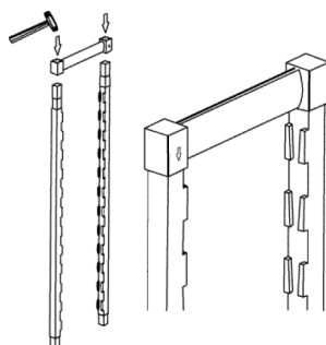
MONTERING AV DET ÖVRE STOLPBESELAGET
