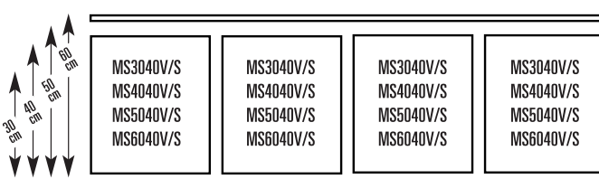
Disposición para traviesas de 160 cm
