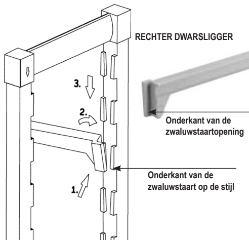
BEVESTIGING VAN DE DWARSLIGGER OP DE STIJL
