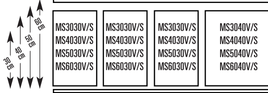
Innordning for 150 cm tverrstenger
