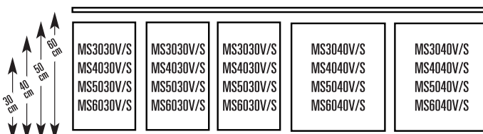
Arrangemang för 170 cm-tvärstag
