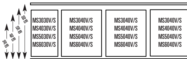
Configurazione del ripiano per la traversa da 170 cm
