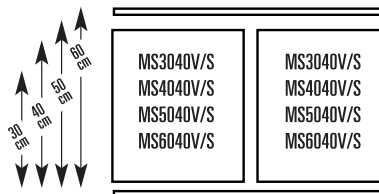
Arrangemang för 110 cm-tvärstag
