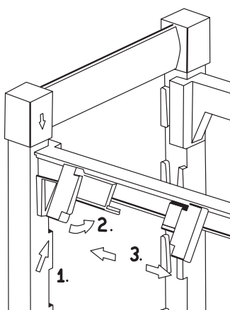
SCHNAPPVERBINDUNGEN DER QUERSTREBE
