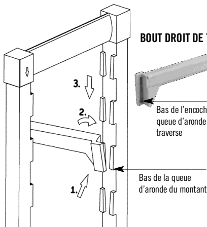
MONTAGE DES TRAVERSES
