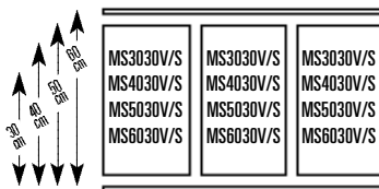
Configuration pour traverse de 120 cm
