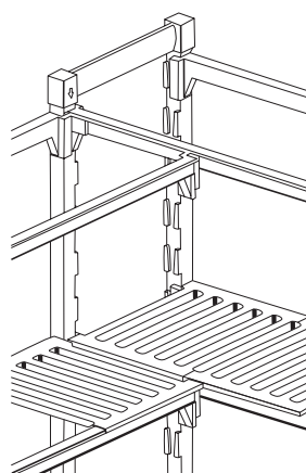
BEFESTIGUNG DER QUERSTREBEN
