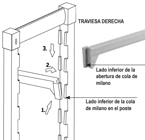
SUJECIÓN DE LAS TRAVIESAS EN LOS POSTES
