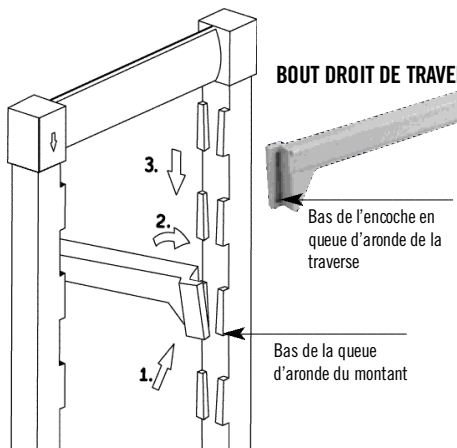
MONTAGE DES TRAVERSES
