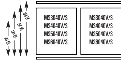
Arrangemang för 110 cm-tvärstag
