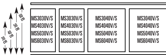
Anordnung für 160-cm-Querstreben
