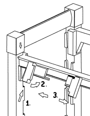
INSÉRER ET ENGAGER LE RACCORD SUR LE BORD DE LA TRAVERSE
