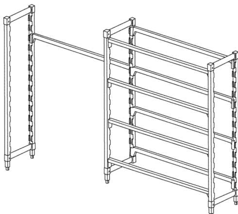
AANBRENGEN VAN DE AANBOUWUNIT
