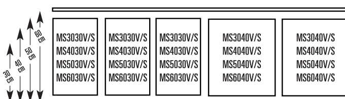
Indeling voor dwarsliggers van 170 cm
