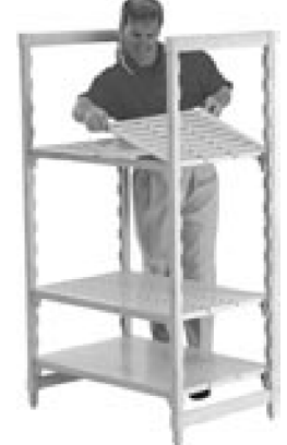
PLAATSING VAN DE SCHAPPEN OP DE DWARSLIGGERS
