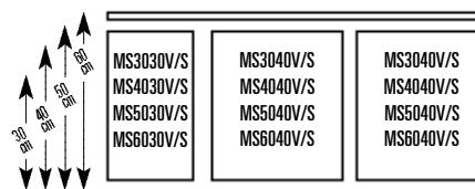
Configuration pour traverse de 130 cm
