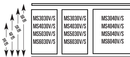
Configurazione del ripiano per la traversa da 100 cm
