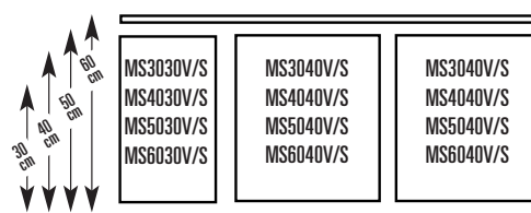
Configurazione del ripiano per la traversa da 130 cm
