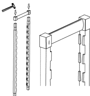
FIJACIÓN DE LA UNIÓN DE POSTES SUPERIOR
