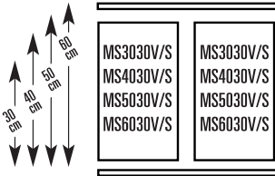
Innordning for 90 cm tverrstenger
