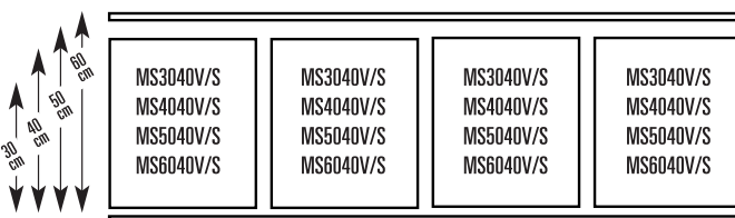
Arrangemang för 160 cm-tvärstag
