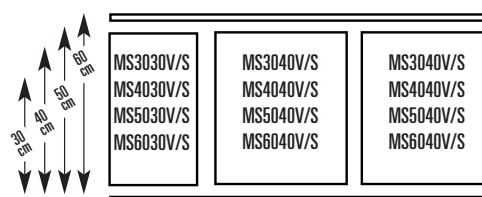
Anordnung für 130-cm-Querstreben
