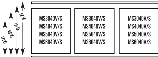
Indeling voor dwarsliggers van 120 cm
