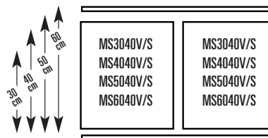
Anordnung für 110-cm-Querstreben
