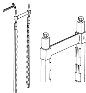
MONTERING AV DET UNDERE STOLPBESELAGET
