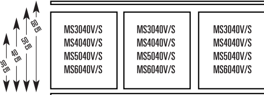
Innordning for 120 cm tverrstenger
