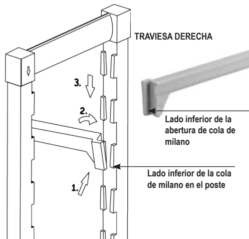
SUJECCIÓN DE LAS TRAVIESAS EN LOS POSTES
