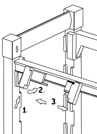
TVÄRSTAGETS SNÄPPLÅS
