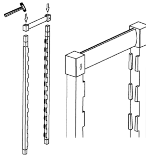
AANBRENGEN VAN DE BOVENSTE STIJLVERBINDING
