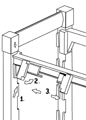
TVÄRSTAGETS SNÄPPLÅS
