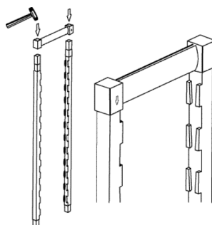
MONTERING AV DET ÖVRE STOLPBESELAGET
