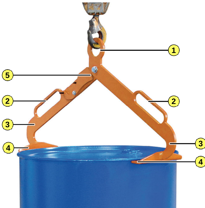
Abb. 3-1: Baugruppen Fasszange Typ LGZ
