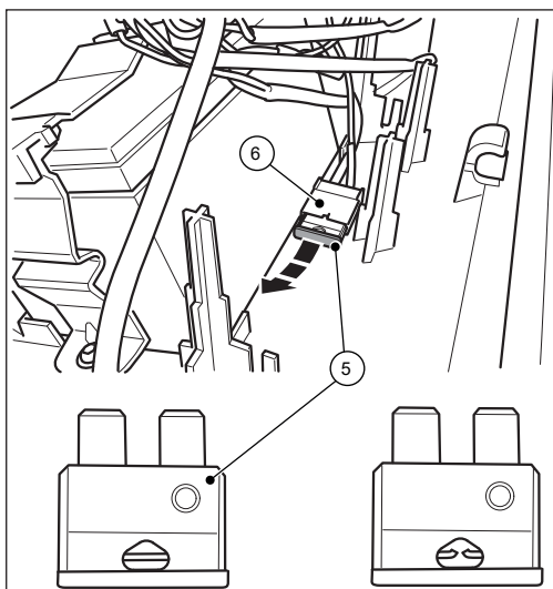
Afb. 20: Zekering F1
