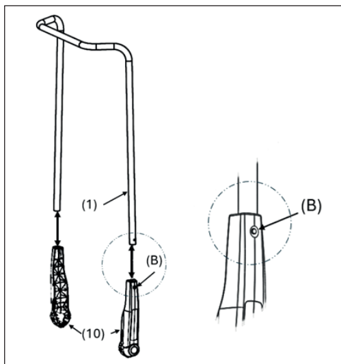
Fig. 8: Montering af håndtagsbeslagene
