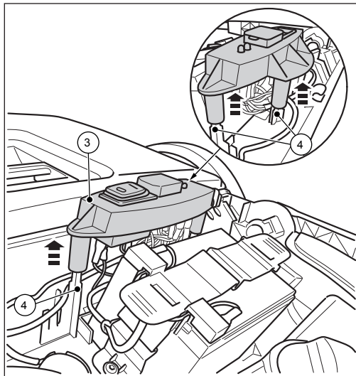
Bild 19: Ta bort omkopplarplattan
