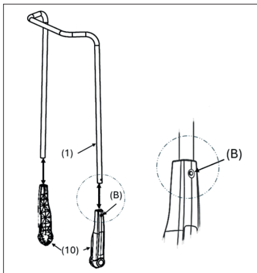
Bild 8: Montera handtagsbeslagen
