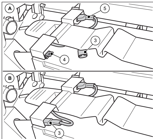
Ábra 10: Akku-csatlakozóvezeték rácsatlakoztatása
