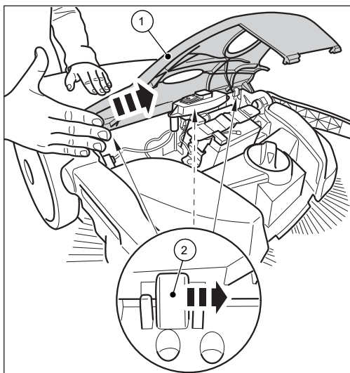
Ábra 18: A burkolat leszerelése
