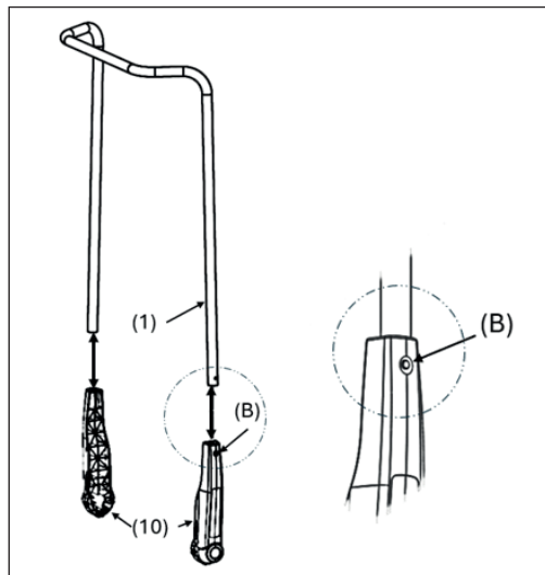
Рис. 8: Монтаж зажимов
