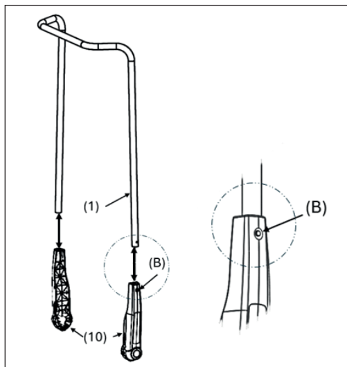
Illustr. 8 : Montage des ferrures de poignée
