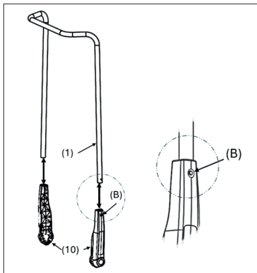
Rys. 8: Montaż uchwytu
