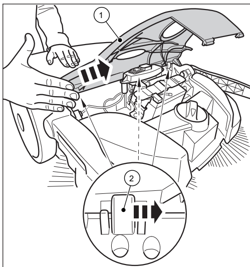
Рис. 18: Снятие кожу
