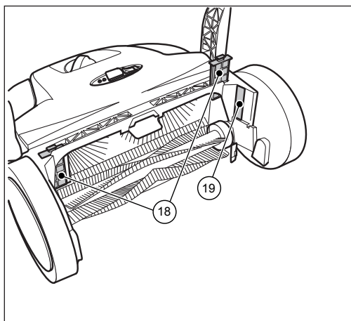
Abb. 3: Komponentenübersicht 3
