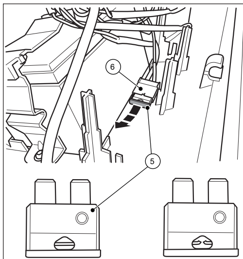
Kuva 20: Sulake F1
