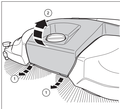
Ábra 9: A burkolat kinyitása
