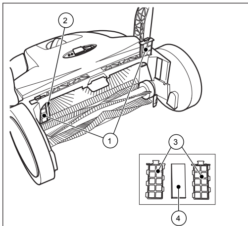
Kuva 21: Pölysuodattimen poistaminen
