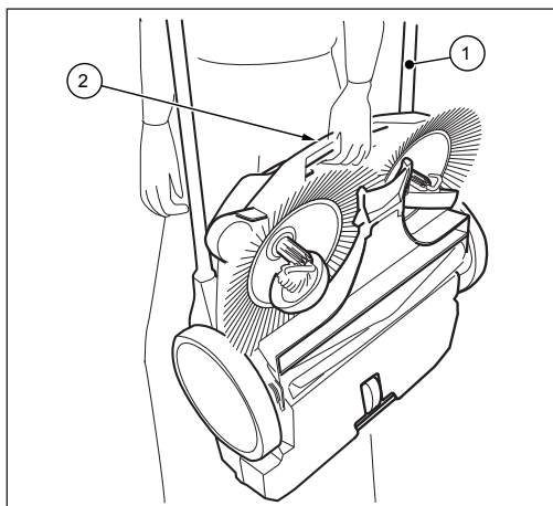
Fig. 7: Bær enheden
