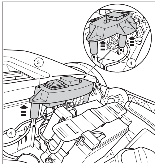
Fig. 19: Demonter bryterplaten
