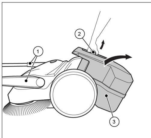
Ábra 17: A hulladéktartály kiürítése
