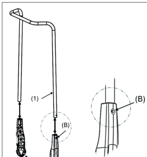
Fig. 8: Montar las guarniciones de manillar
