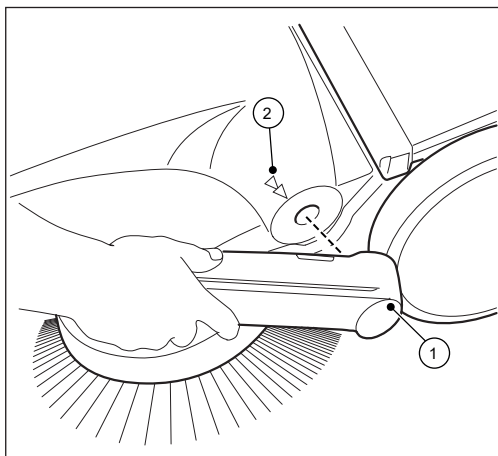
Afb. 22: Demontage van de duwbeugel
