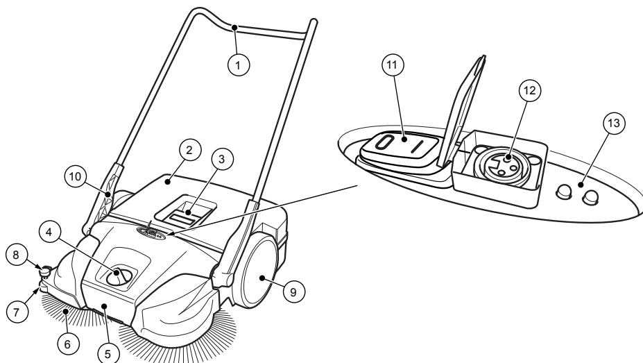
Obr. 1: Přehled součástí
