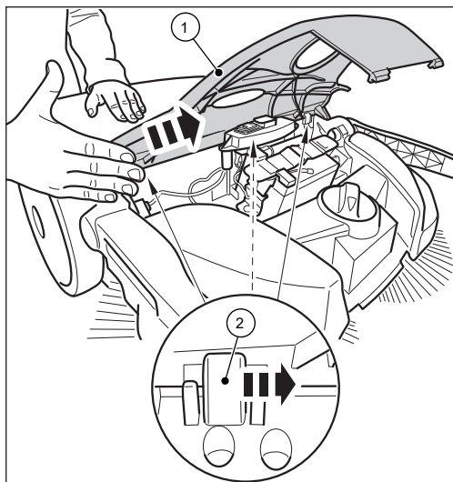
Fig. 18: Demonter dekslet
