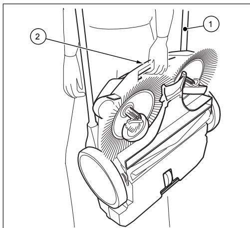
Obr. 7: Přenášení stroje
