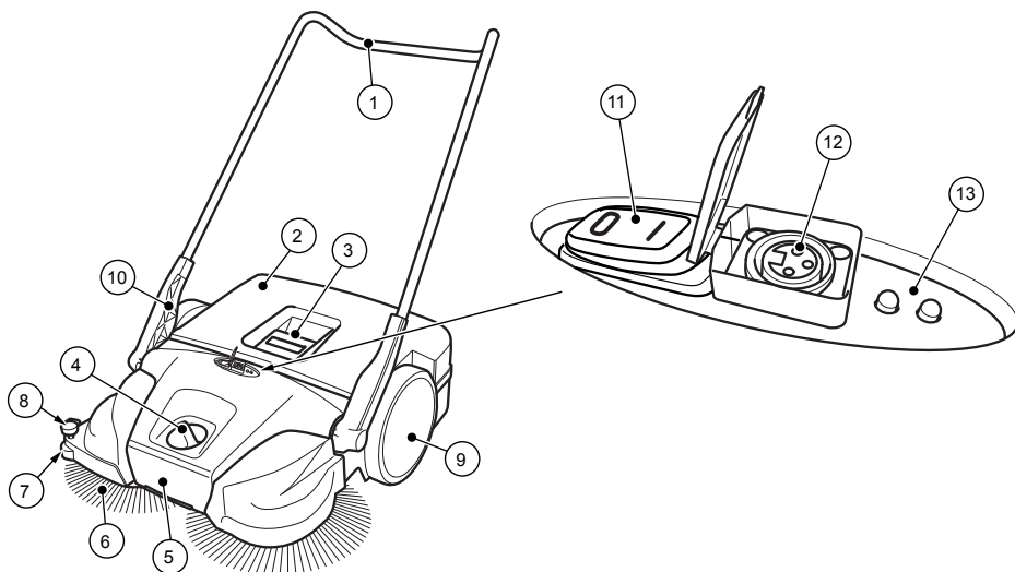
Abb. 1: Komponentenübersicht 1
