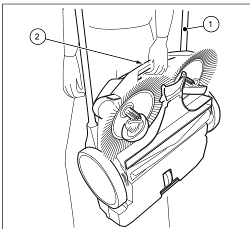
Bild 7: Bära maskinen
