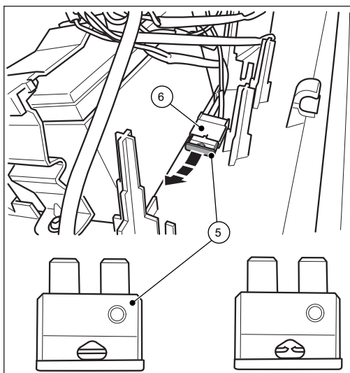
Fig. 20: Fuse F1
