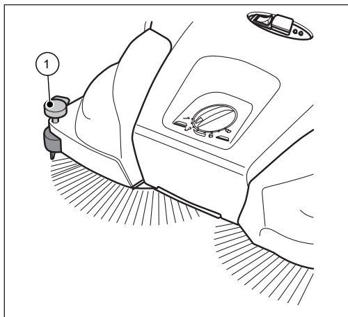
Obr. 14: Nastavení přidržovače
