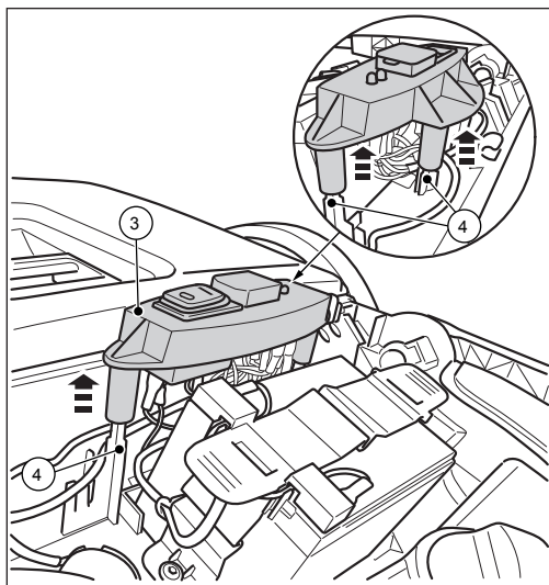
Ábra 19: Kapcsolólap kiszerelése
