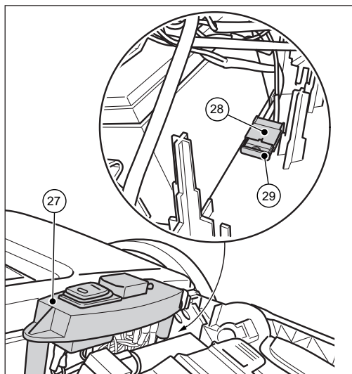
Bild 6: Översikt över komponenter 6
