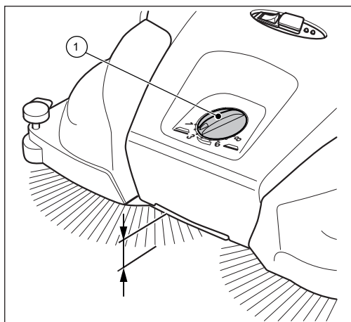
Fig. 13: Regolazione in altezza delle scope laterali
