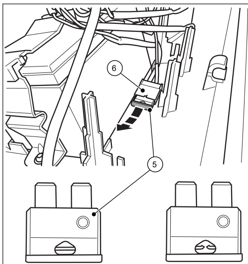
Ábra 20: F1 biztosíték
