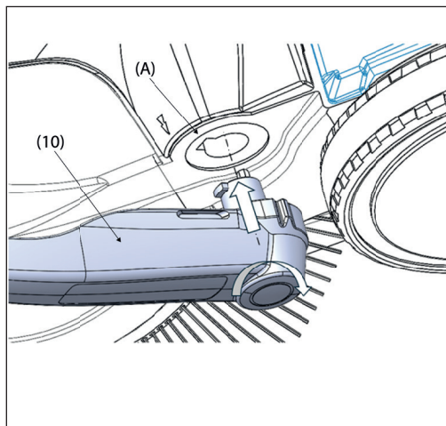
Abb. 9: Haube öffnen
