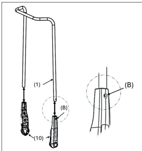
Afb. 8: Montage van de handgrepen
