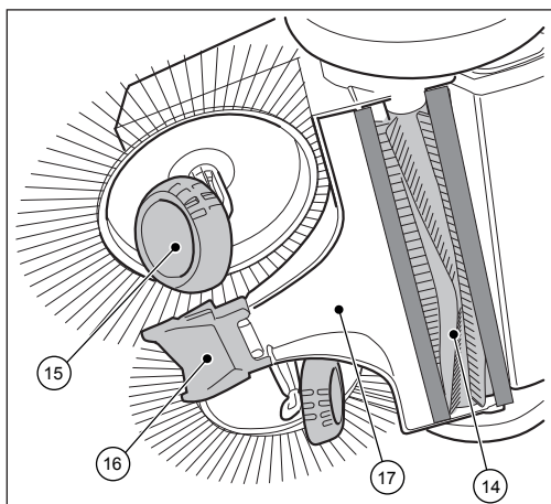
Obr. 2: Přehled součástí 2
