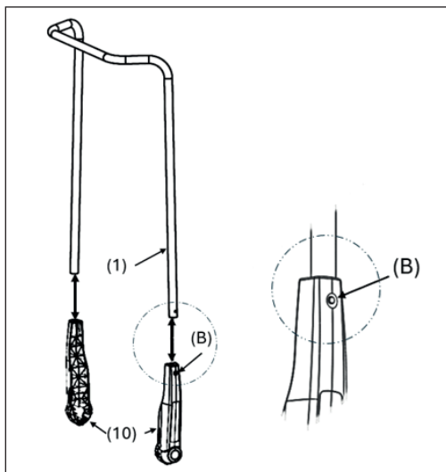
Obr. 8: Montáž kování držadla
