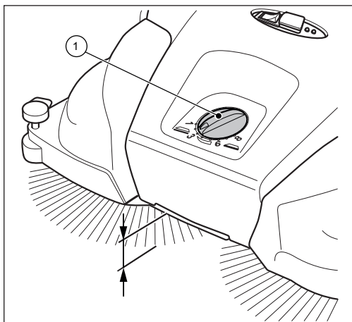
Obr. 13: Nastavení výšky talířových kartáčů
