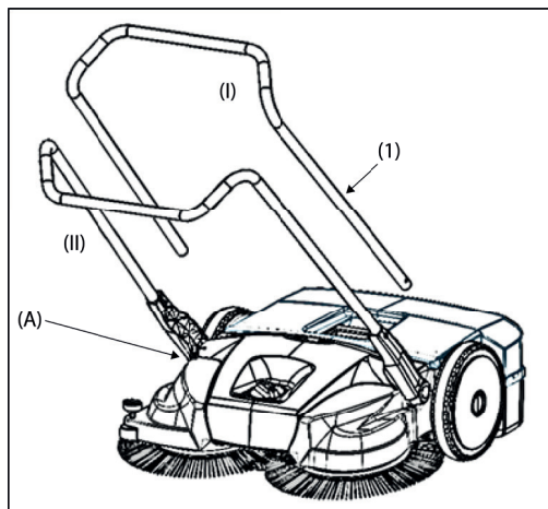
Obr. 9: Otevření krytu
