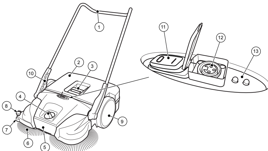
Afb. 1: Componentenoverzicht 1
