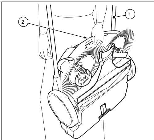
Kuva 7: Laitteen kantaminen
