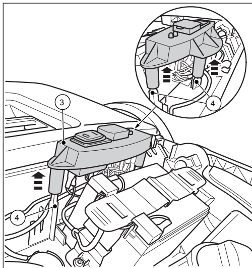
Kuva 19: Kytkeinlevyn irrottaminen
