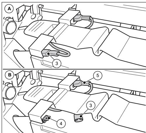
Abb. 24: Akku-Anschlussleitung abklemmen
