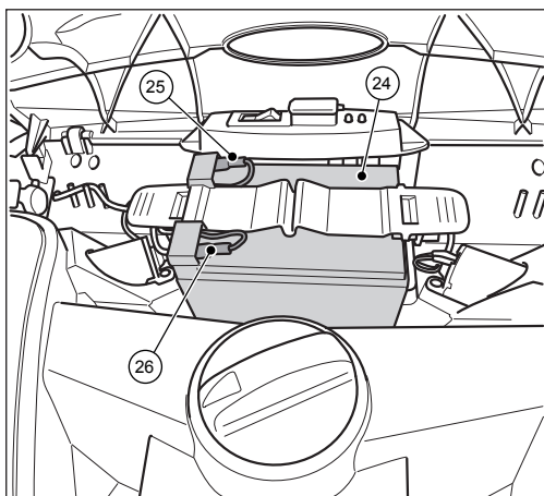
Kuva 5: Laitteen osat 5
