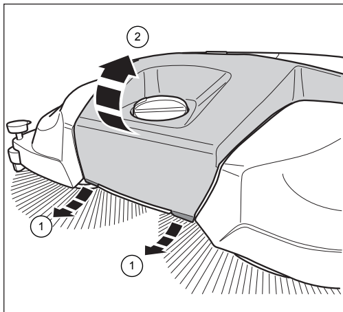
Obr. 9: Otevření krytu
