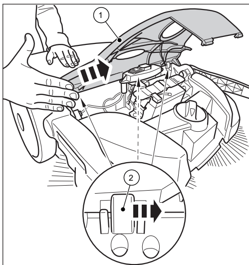
Fig. 18: Desmontaje de la cubierta
