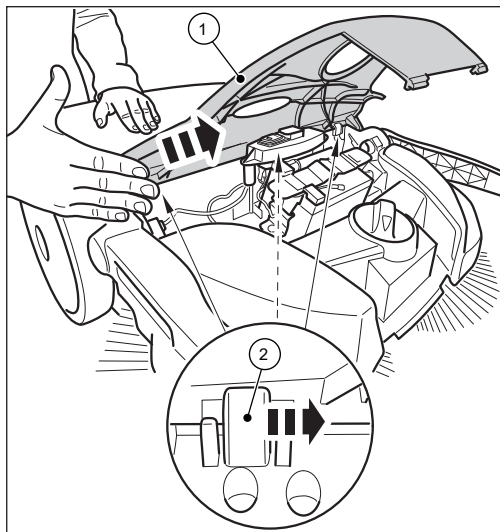
Abb. 18: Haube ausbauen
