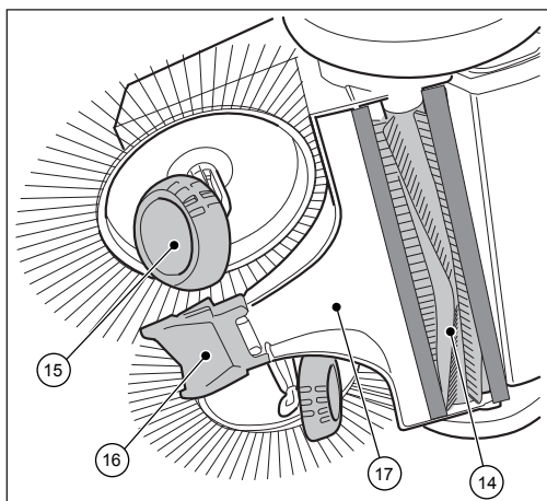
Abb. 2: Komponentenübersicht 2
