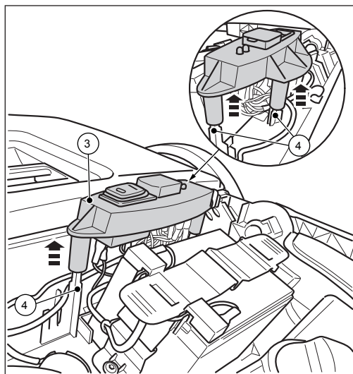
Rys. 19: Demontaż płytki przełącznika
