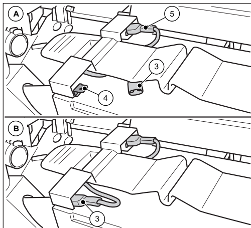
Afb. 10: Accu-aansluitkabel aansluiten
