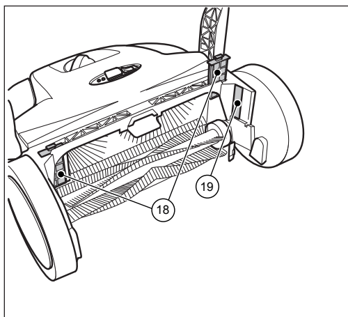
Kuva 3: Laitteen osat 3
