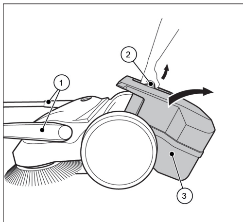
Kuva 17: Säiliön tyhjentäminen
