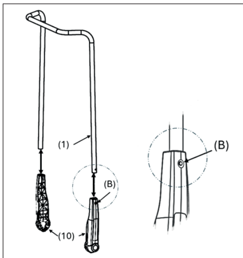
Kuva 8: Kahvan helojen asennus
