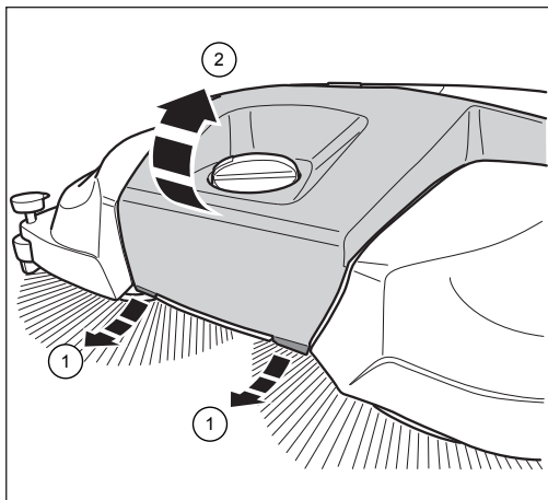
Afb. 9: Kap openen
