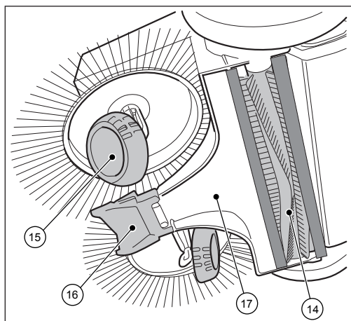
Rys. 2: Przegląd komponentów 2
