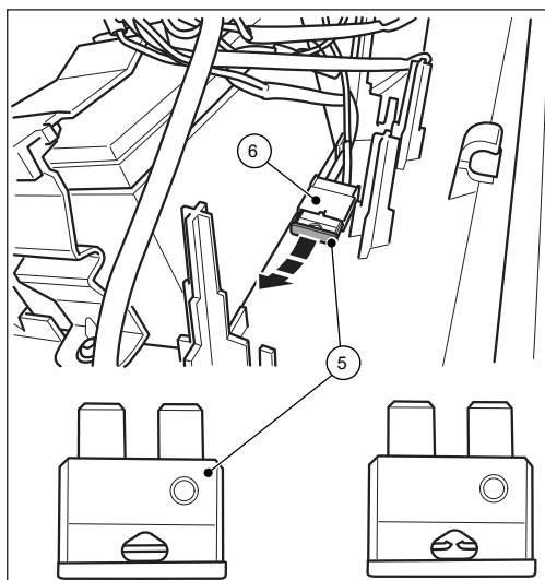
Fig. 20: Fusibile F1
