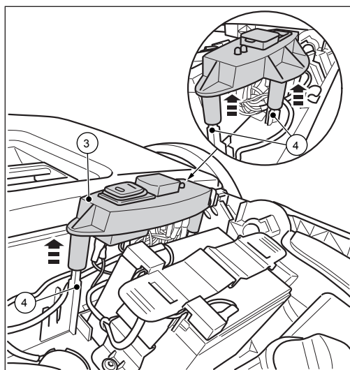
Afb. 19: Schakelplaat uitbouwen
