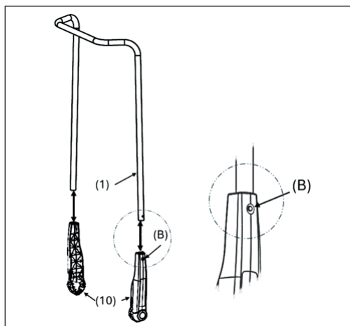
Abb. 8: Griffbeschläge montieren
