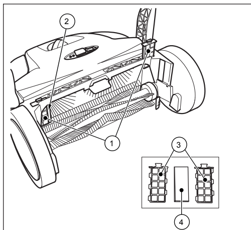
Ábra 21: A porszűrő kiserelése
