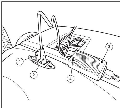
Kuva 11: Liitä laturi
