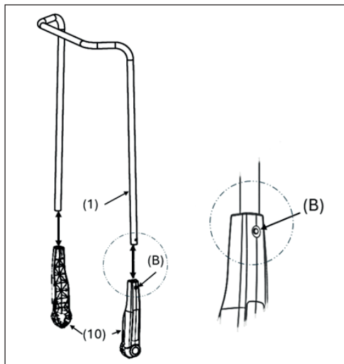
Fig. 8: Montaggio dei braccetti dell'archetto
