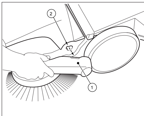
Fig. 14: Smontaggio dell'archetto di spinta
