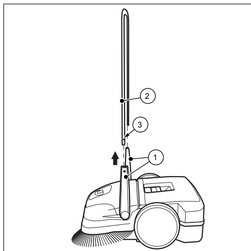
Fig. 13: Smontaggio dell'archetto di spinta (non starmix 497)
