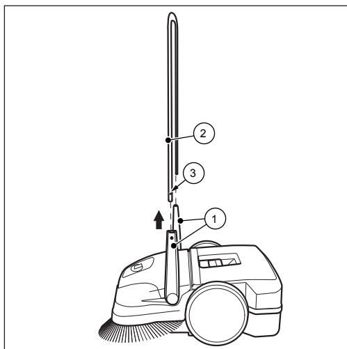
Abb. 13: Schiebebügeldemontage (nicht starmix 497)
