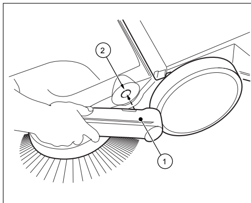
Fig. 7: Montaggio braccetti dell'archetto
