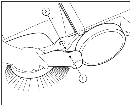
Abb. 14: Schiebebügeldemontage
