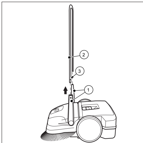
Fig. 13: Demontering af skubbebøjle (ikke starmix 497)
