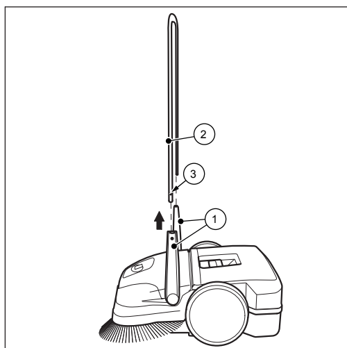
Рис. 13: Демонтаж дугообразной ручки («не starmix 497»)
