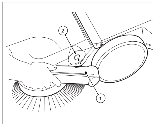
Fig. 7: Montaje de las guarniciones de manillar
