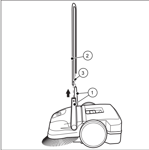
Şek. 13: İtme kolunun söküm işlemi (starmix 497 değil)
