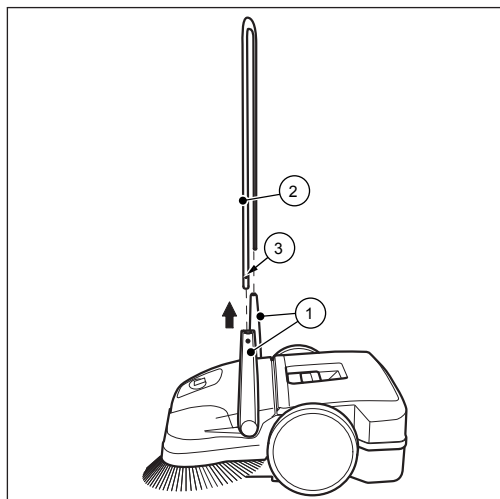
Rys. 13: Demontaż uchwyty do przesuwania (nie starmix 497)
