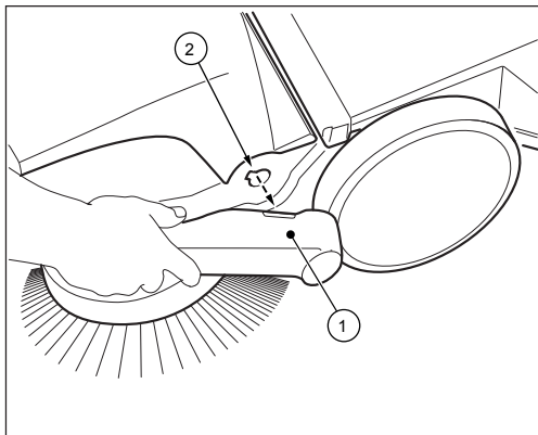
Illustration 14 : Démontage de l'arceau rétractable
