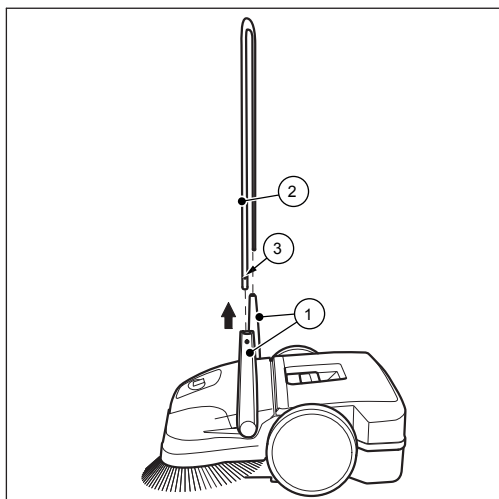
Kuva 13: Työntöaisan irrottaminen (ei starmix 497)
