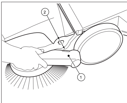
Bild 14: Nedmontering av skjutbygeln
