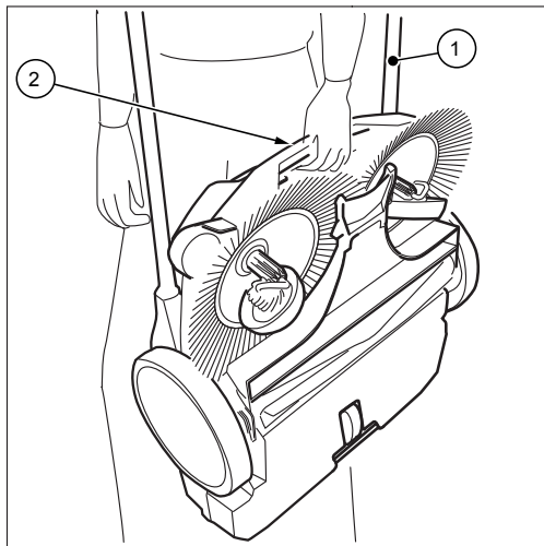
Fig. 6: Trasportare l'apparecchio
