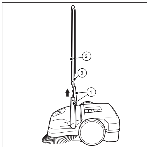
Fig. 13: Desmontaje del manillar (no starmix 497)
