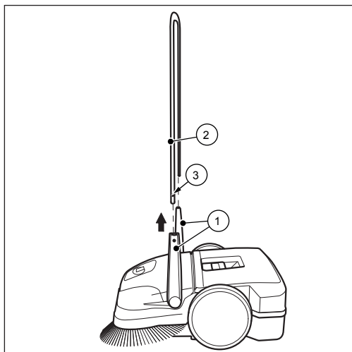
Fig. 13: Desmontagem do varão de empurrar (não starmix 497)
