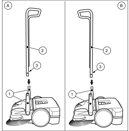
Şek. 8: İtme kolu montajı
