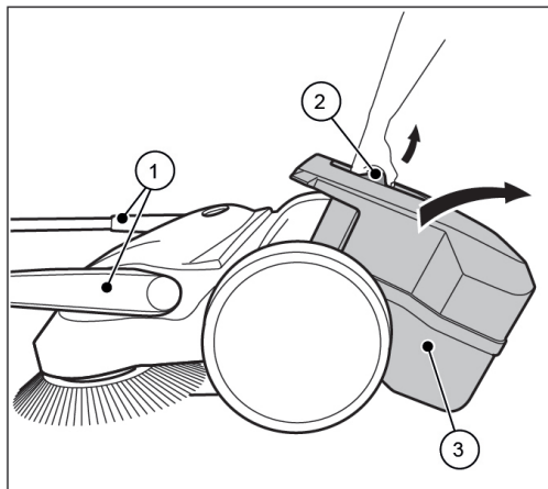
Fig. 11: Affaldsbeholderen tømme
