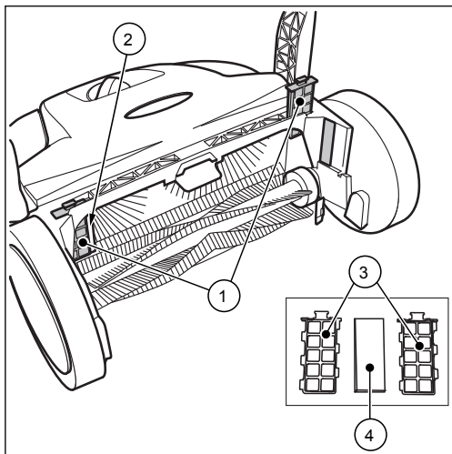
Abb. 12: Staubfilterentnahme
