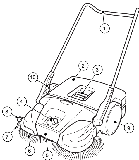
Abb. 1: Komponentenübersicht 1
