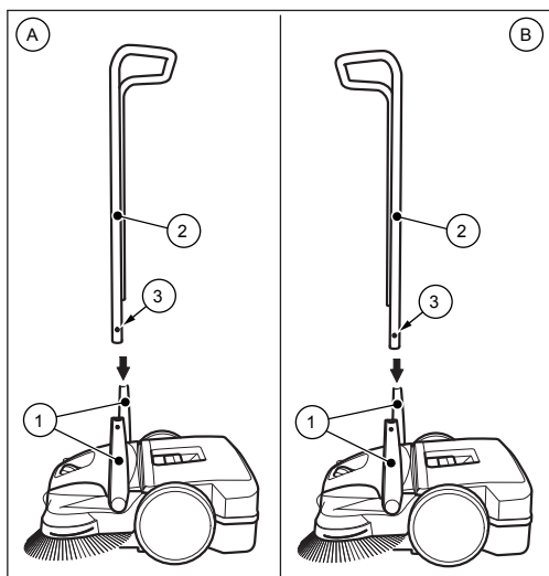
Afb. 8: Duwbeugelmontage
