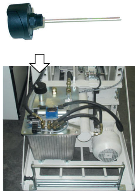
BelüftungsfILTER Art. Nr. 6.116.195.090
