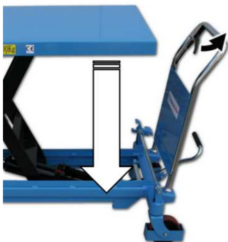
Illustration 10 Nedsænkning
