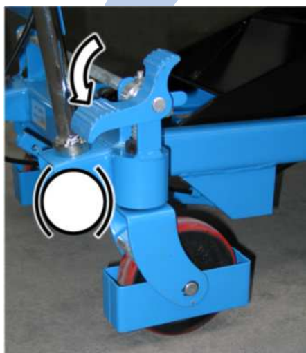
Obrázok 5 Aktivovanie brzdy
