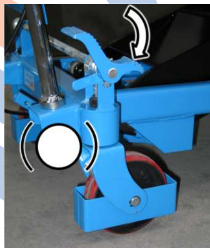
Bilde 6 løsne bremsen
