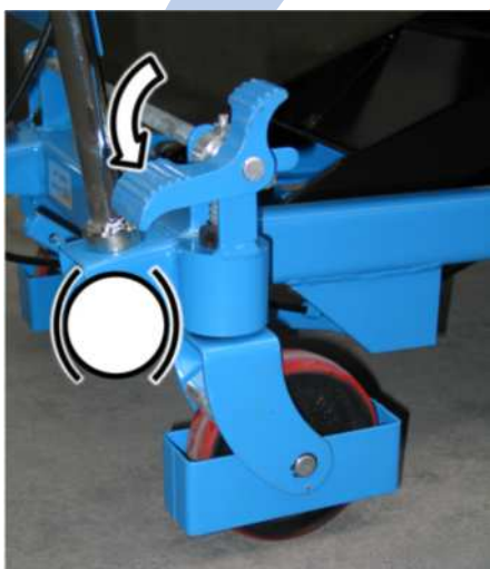
Afbeelding 5 Rem activeren
