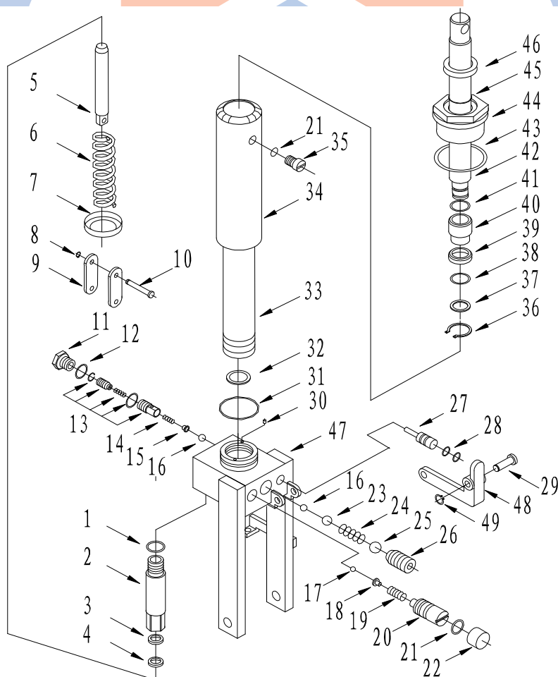
Afbeelding 13 Hydraulica
