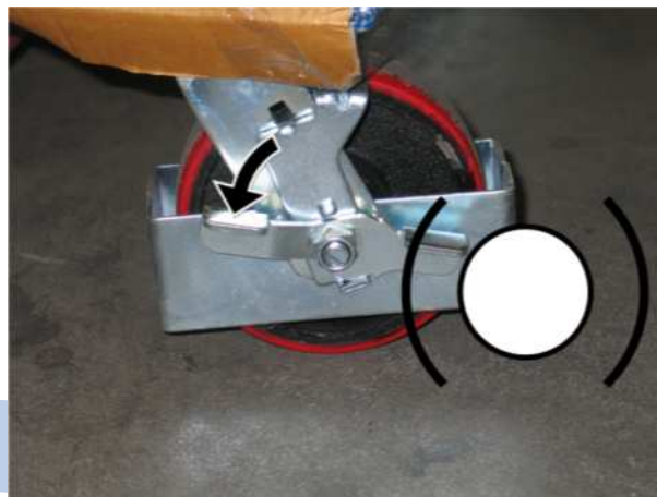
Afbeelding 4 Rem lossen
