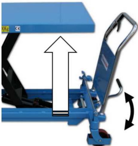
Slika 9 Dviganje
