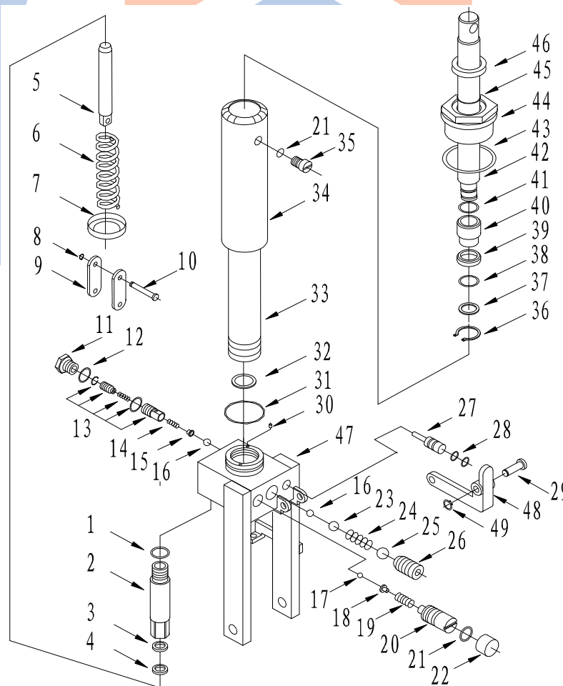
Figura 13 Hidráulica
