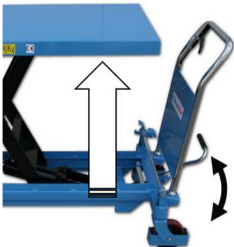
Afbeelding 9 Heffen
