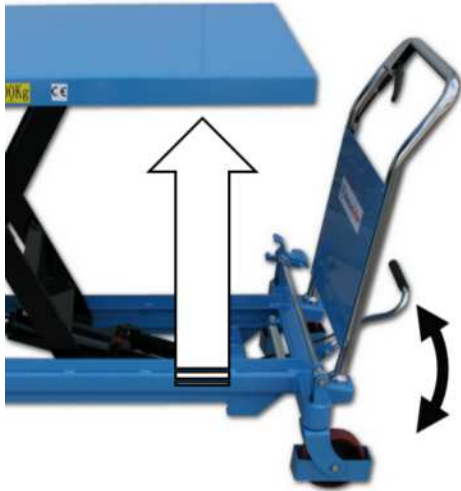
Bilde 9 Heving
