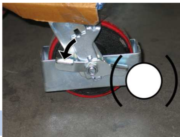
Рисунок 4 Отпускание тормоза
