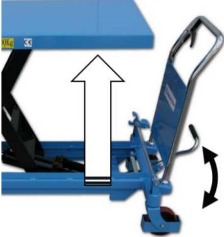
Şekil 9 Kaldırma
